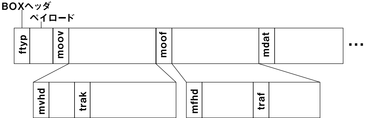
図 4. MP4 の構造
