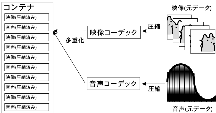
図 3. 動画の構成
