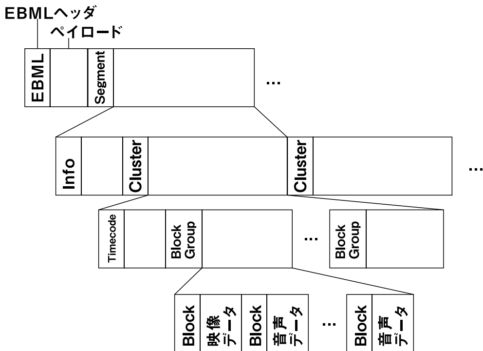
図 7. MKV の構造
