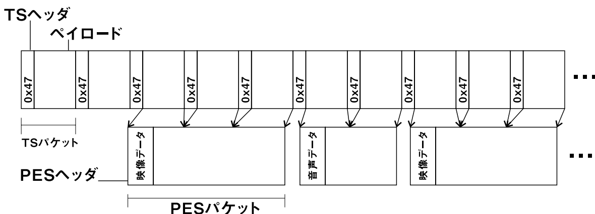
図 6. MPEG-2 TS の構造
