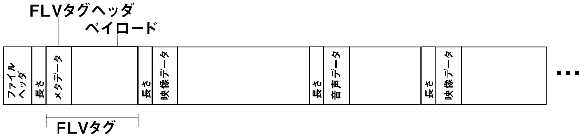
図 8. FLV の構造
